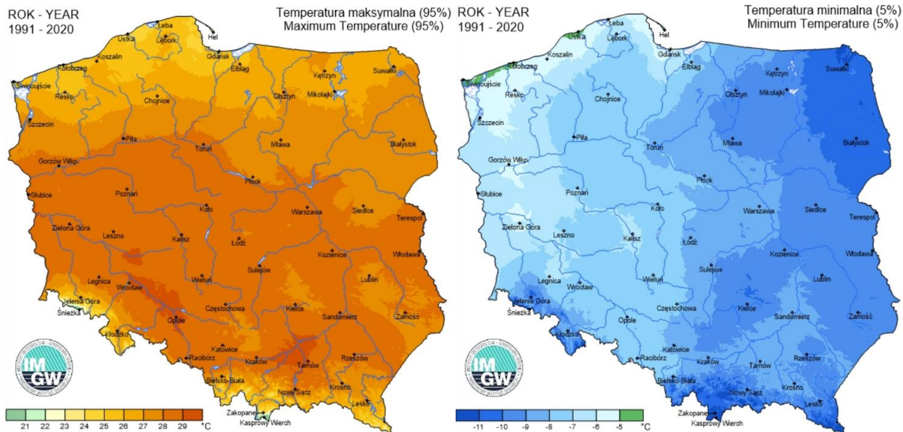
Rysunek 4 Ekstremalne temperatury maksymalne i minimalne w Polsce w latach 1991-2020 r.
